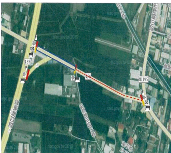
和美鎮美寮路(彰6線)道路拓寬工程-封閉第3工區第1階段交通維持示意圖
