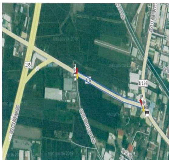
和美鎮美寮路(彰6線)道路拓寬工程-封閉第3工區第2階段交通維持示意圖
